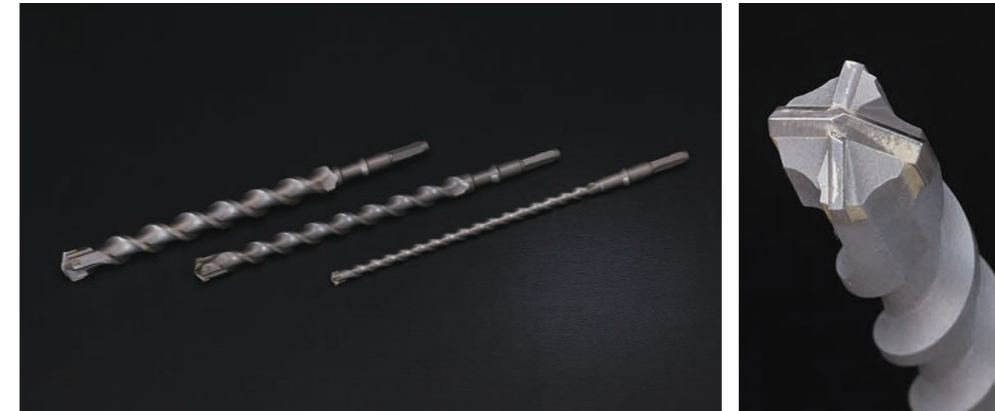
ハンマークロスドリル〈六角軸〉(ロングタイプ) 全長420mm
